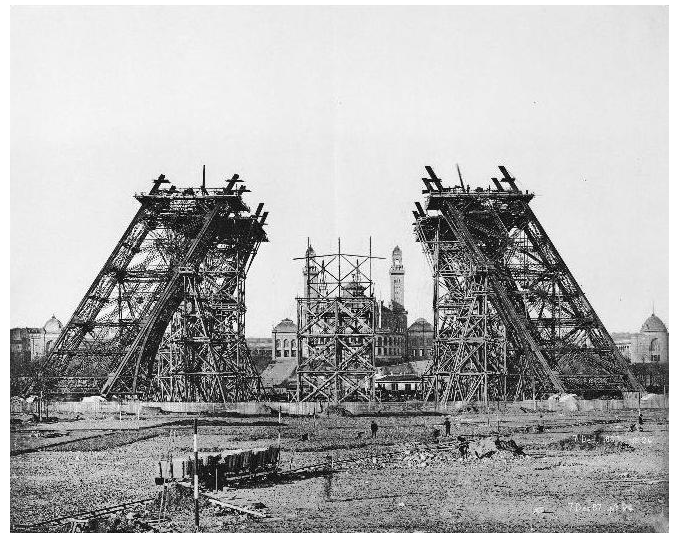
1887: DE MONTAGE VAN EEN STEUNPILAAR VOOR DE BOUW VAN DE EERSTE VERDIEPING
